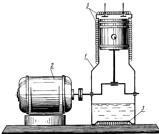
1 — двигатель; 2 — электромотор; 3 — электронагревательные элементы
